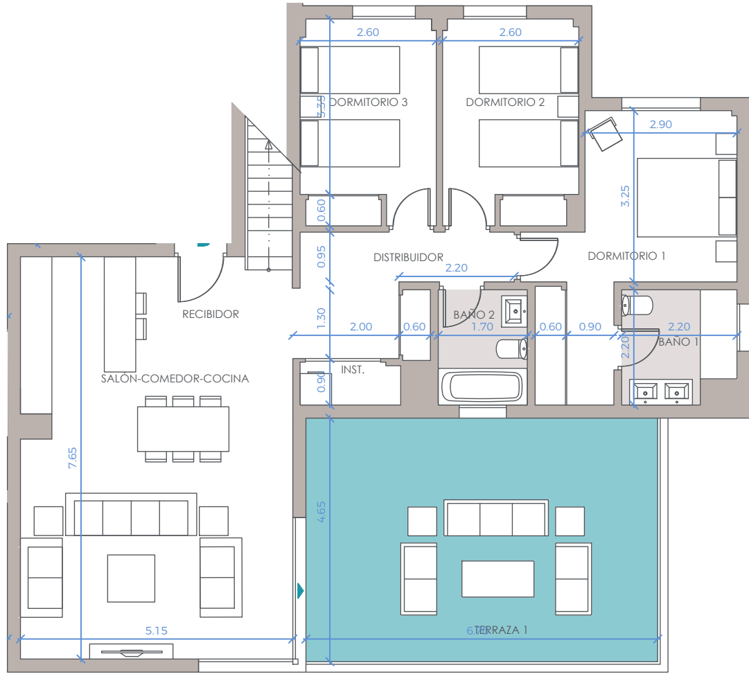
PLANTA SEGUNDA
