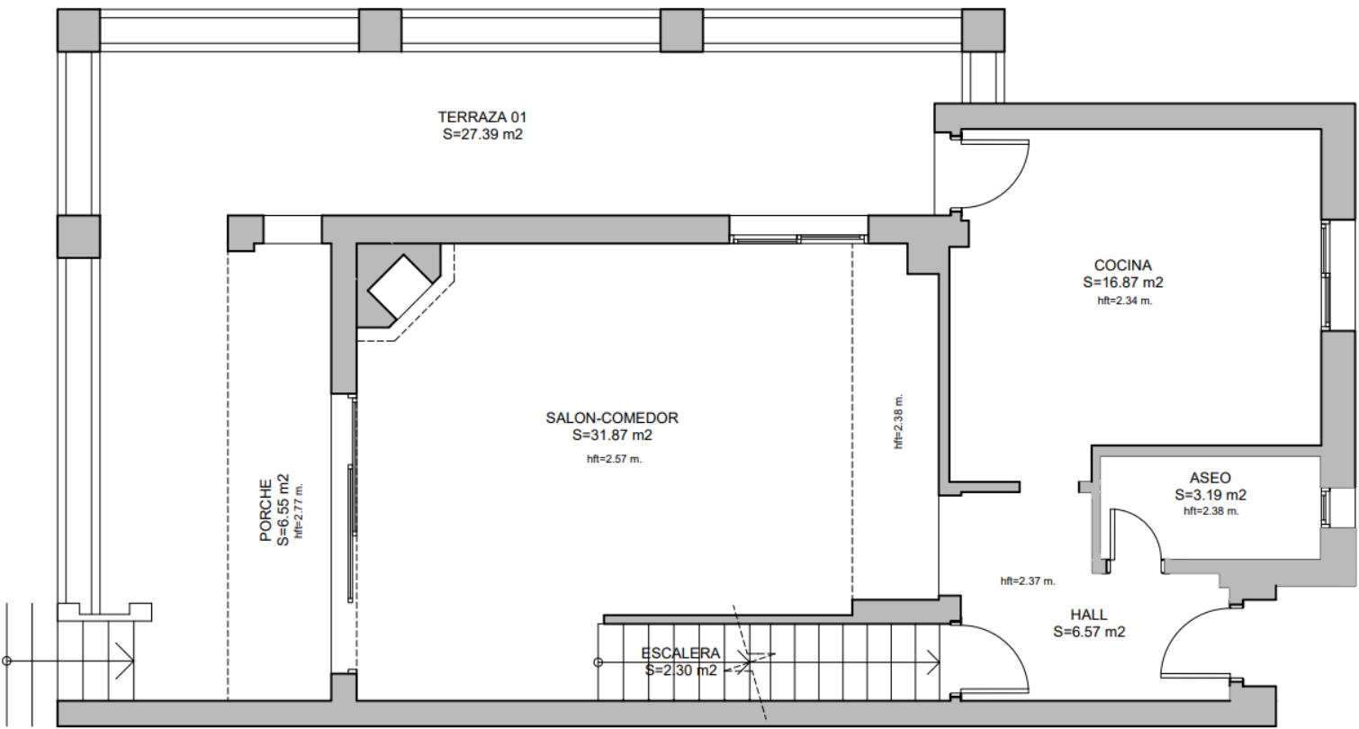
PLANTA BAJA
