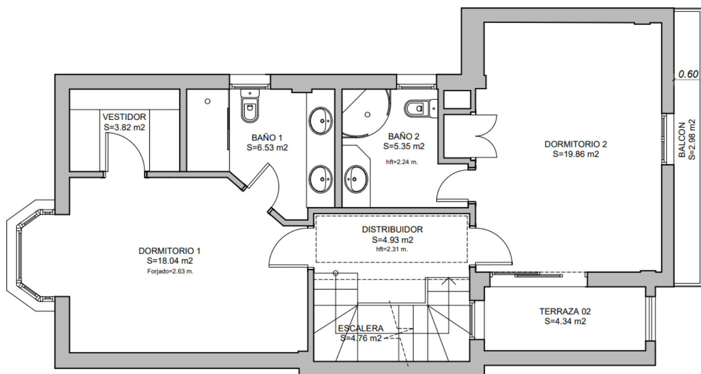
PLANTA PRIMERA
