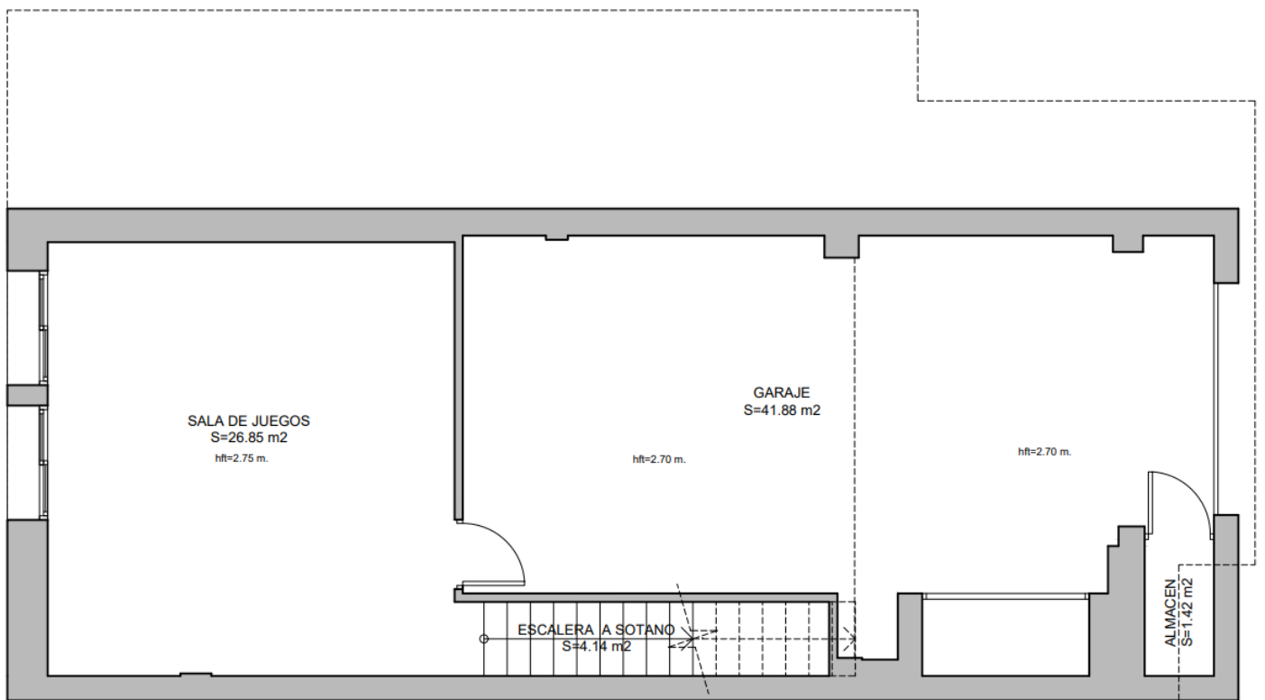
PLANTA SOTANO
