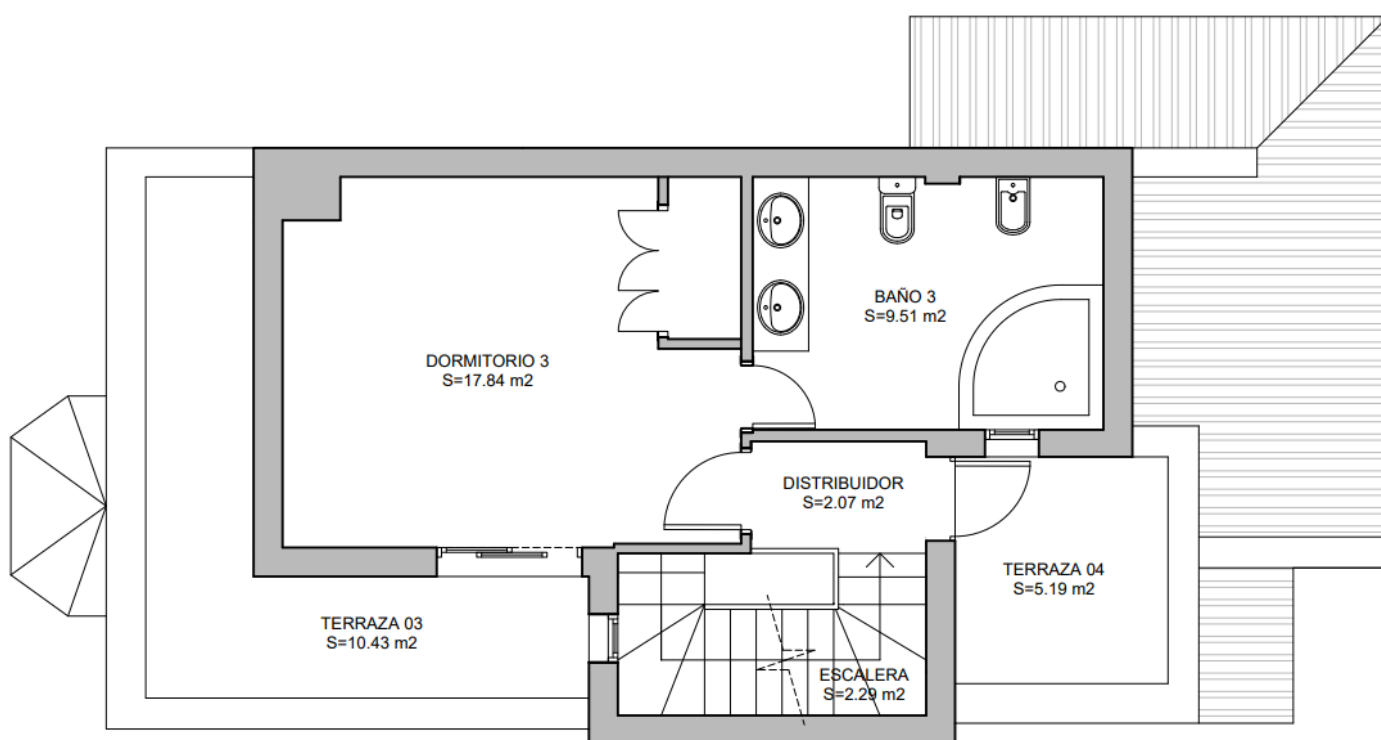
PLANTA BAJOCUBIERTA
