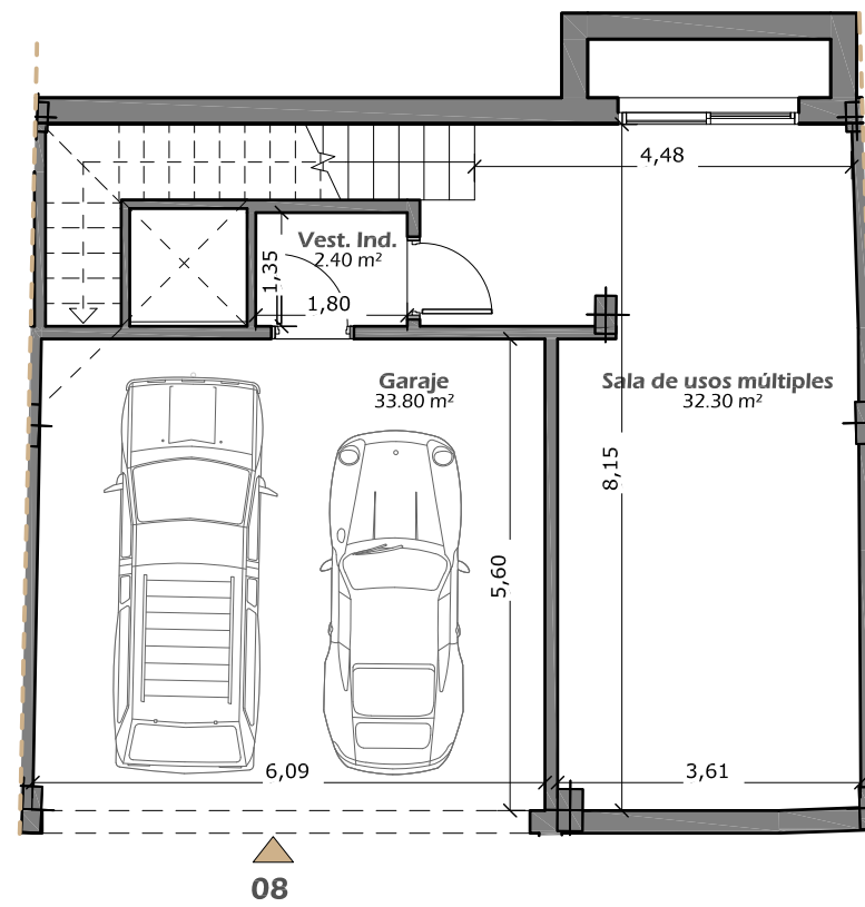
Planta Sótano
