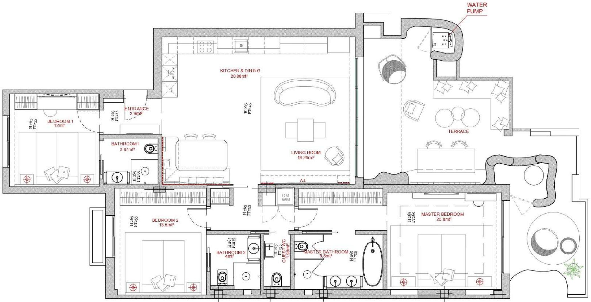
PLAN / PLANTA 1:75
