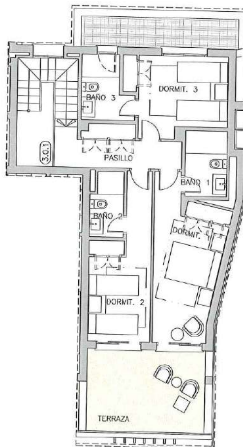
PLANTA PRIMERA
