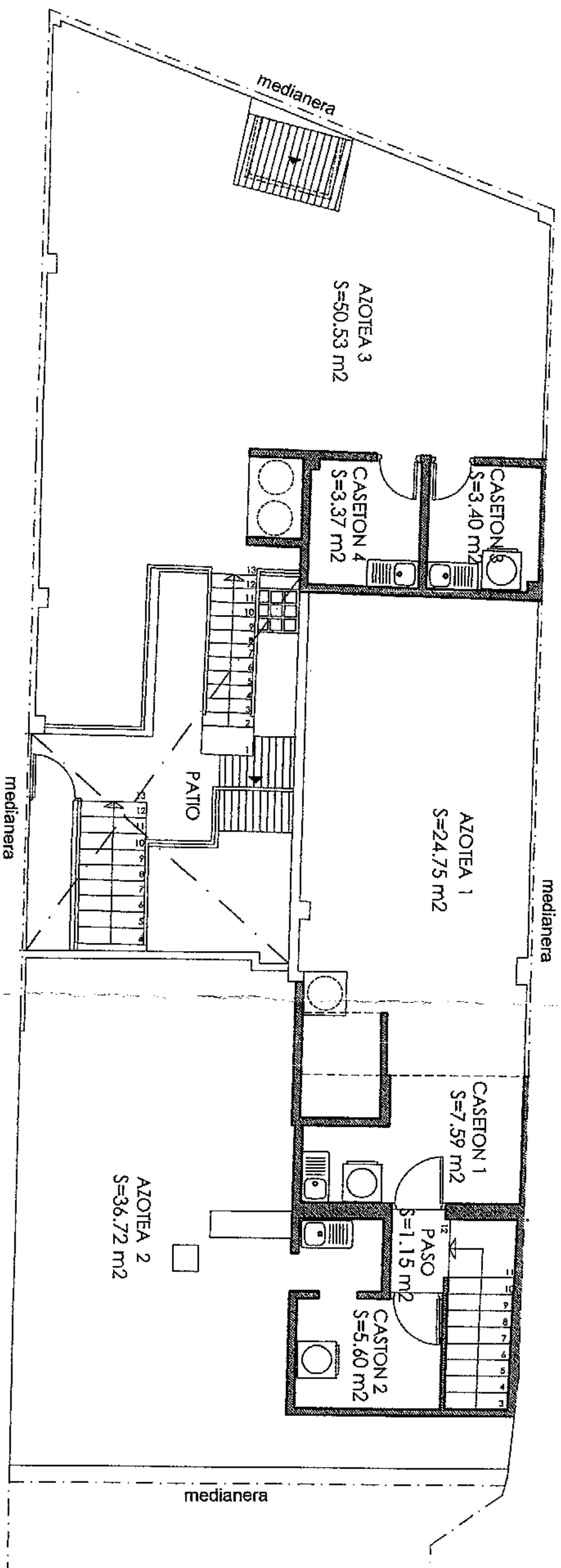
DISTRIBUCIÓN PLANTA AZOTEA
