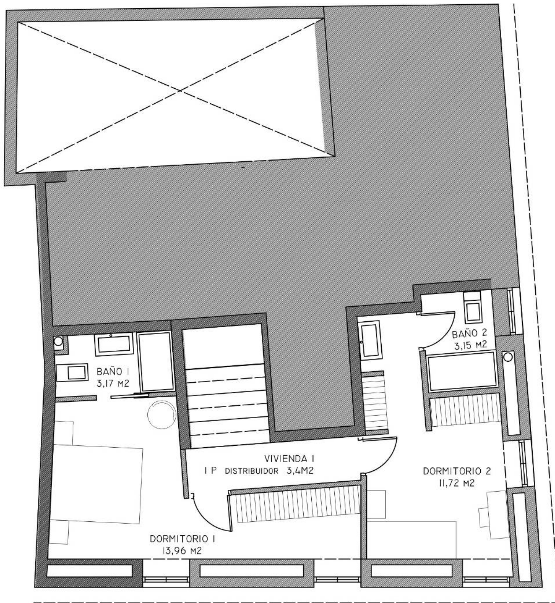
PLANTA PRIMERA
