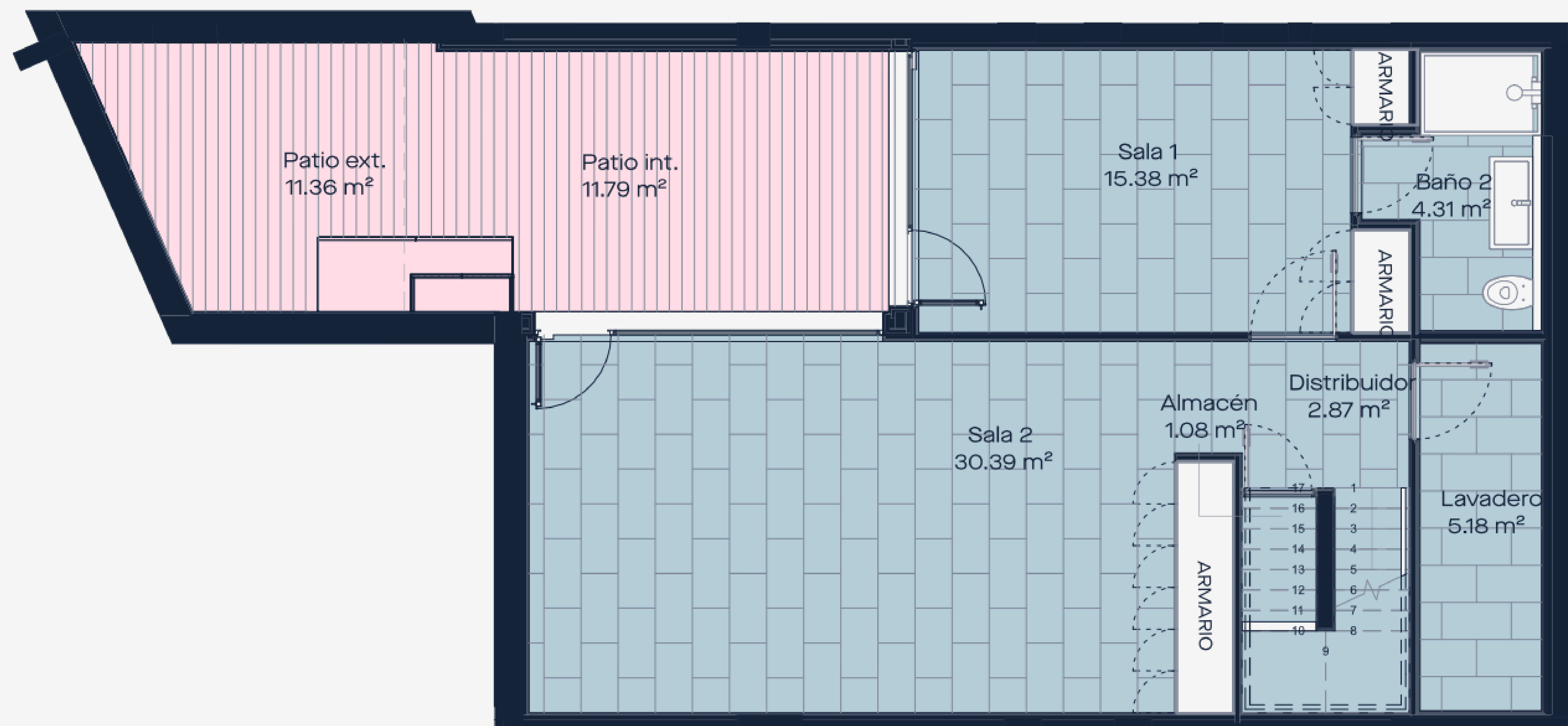
Planta Sótano / BASEMENT FLOOR
