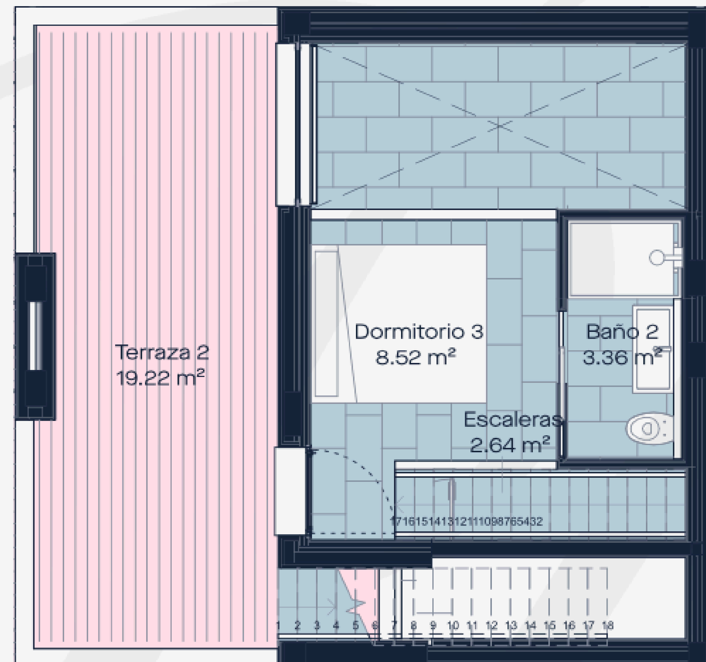
Planta Primera / FIRST FLOOR
