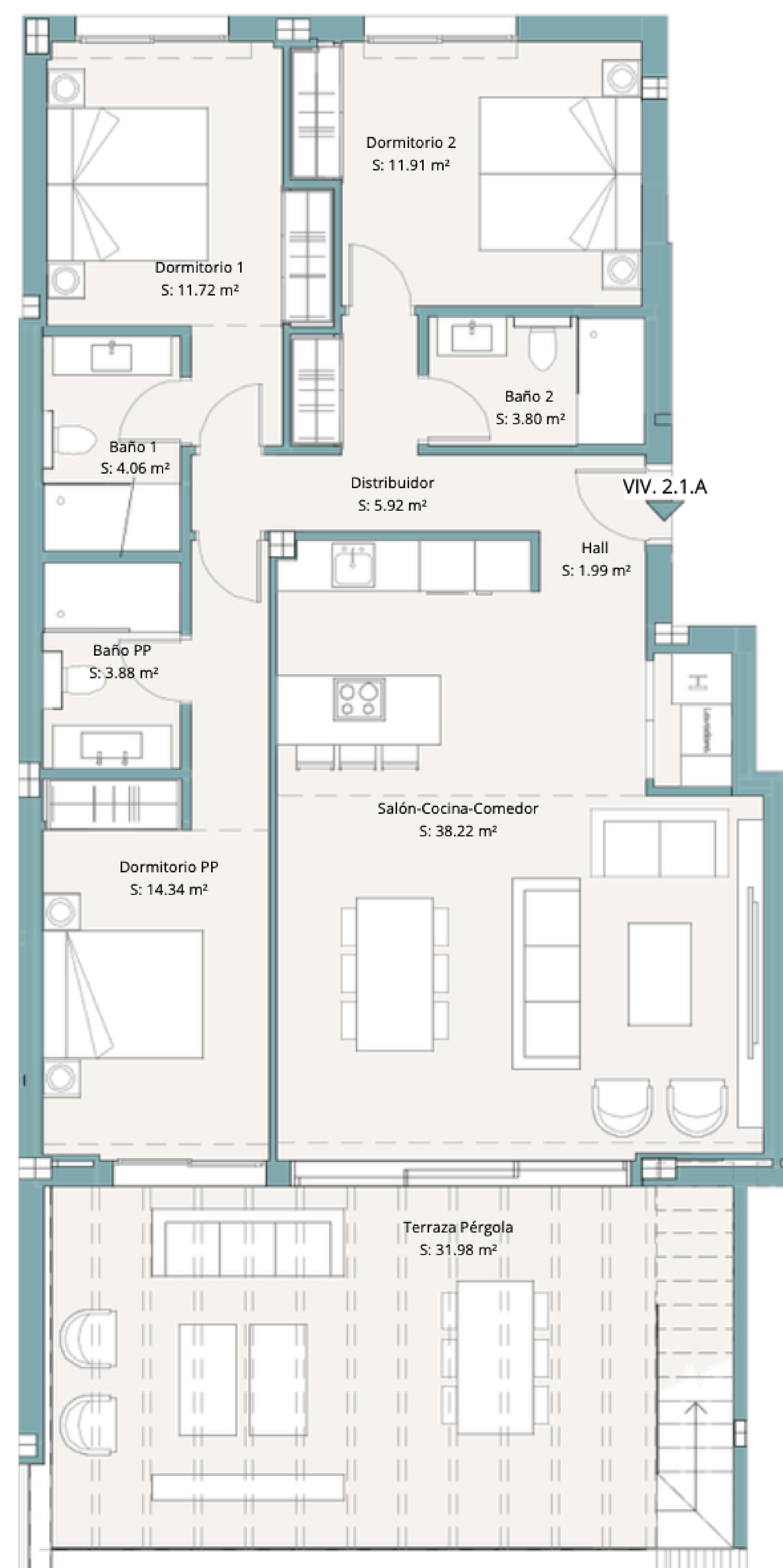
PLANTA PRIMERA
