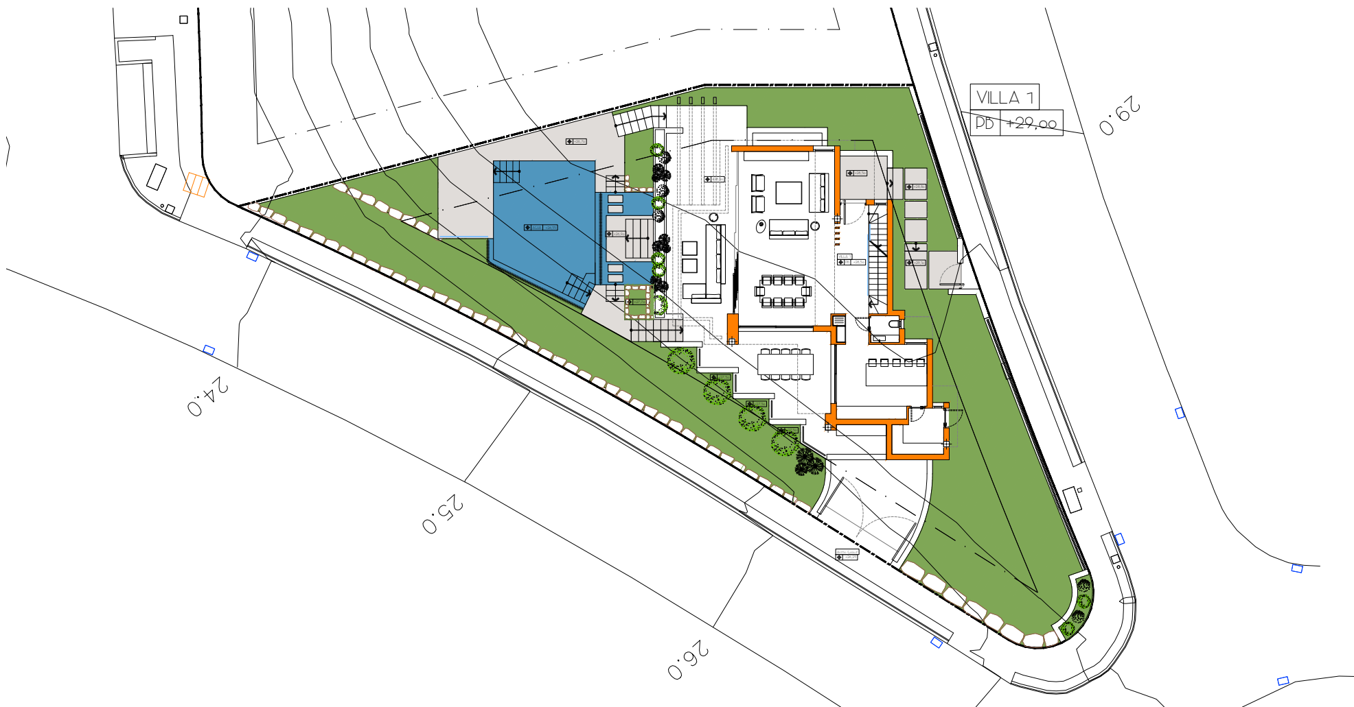
SITE MAP EMPLAZAMIENTO
