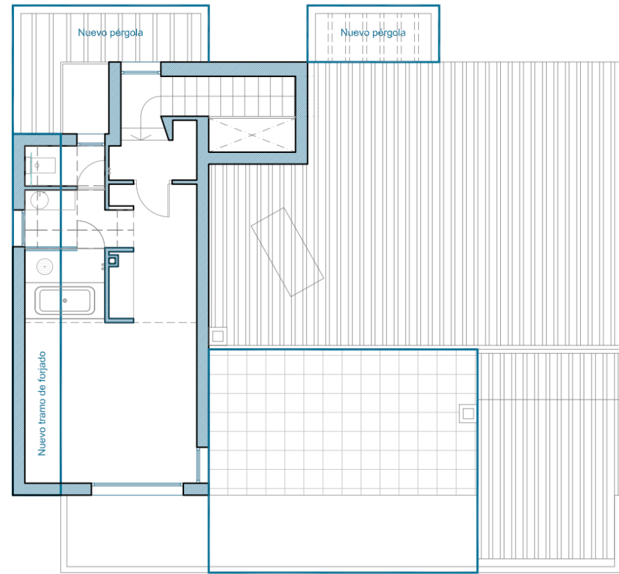
PLANTA PRIMERA
