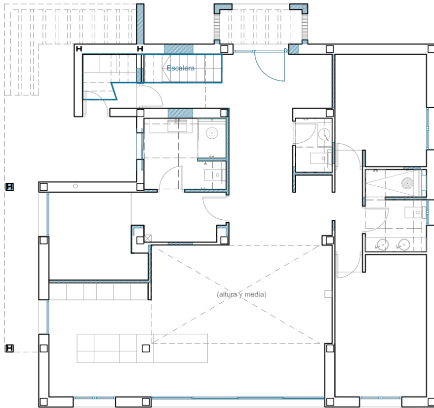
PLANTA BAJA
