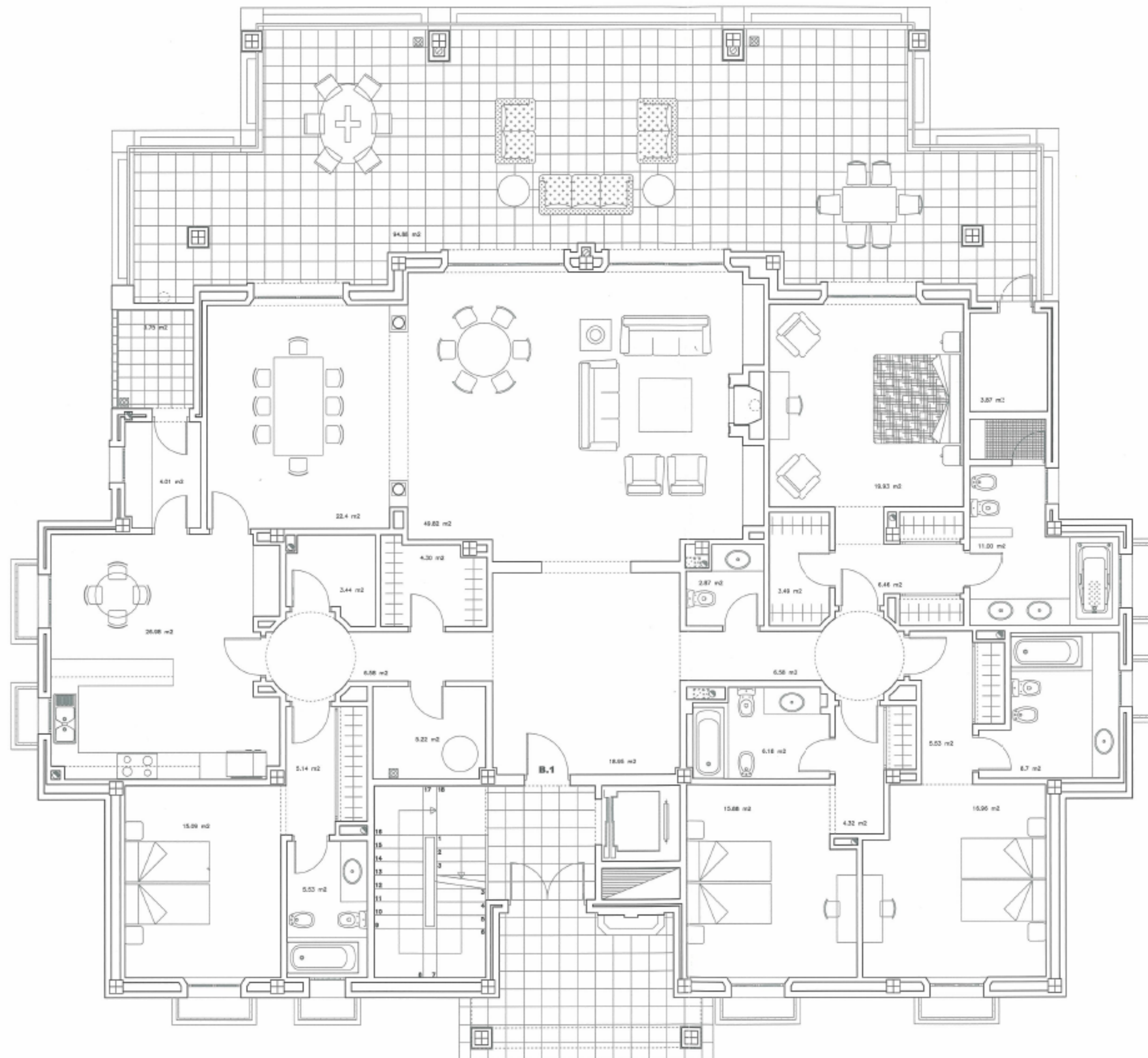
PLANTA BAJA (ACCESO) GROUND FLOOR (ACCESS) E:1/100
