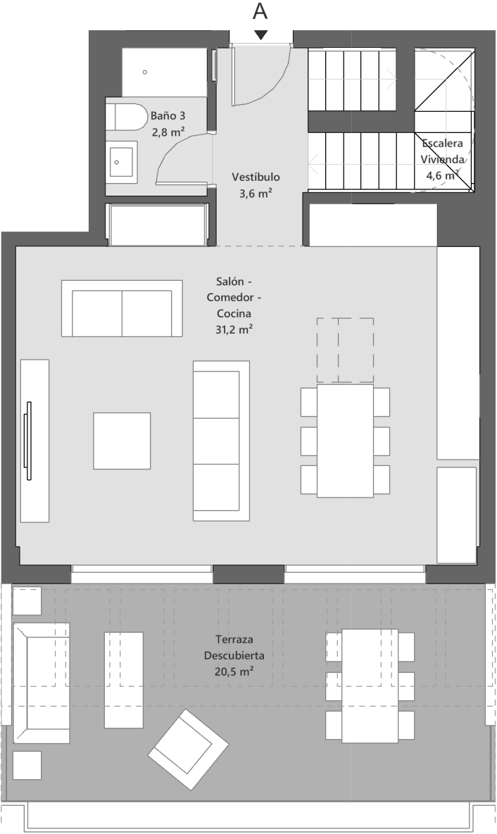
Planta segunda
