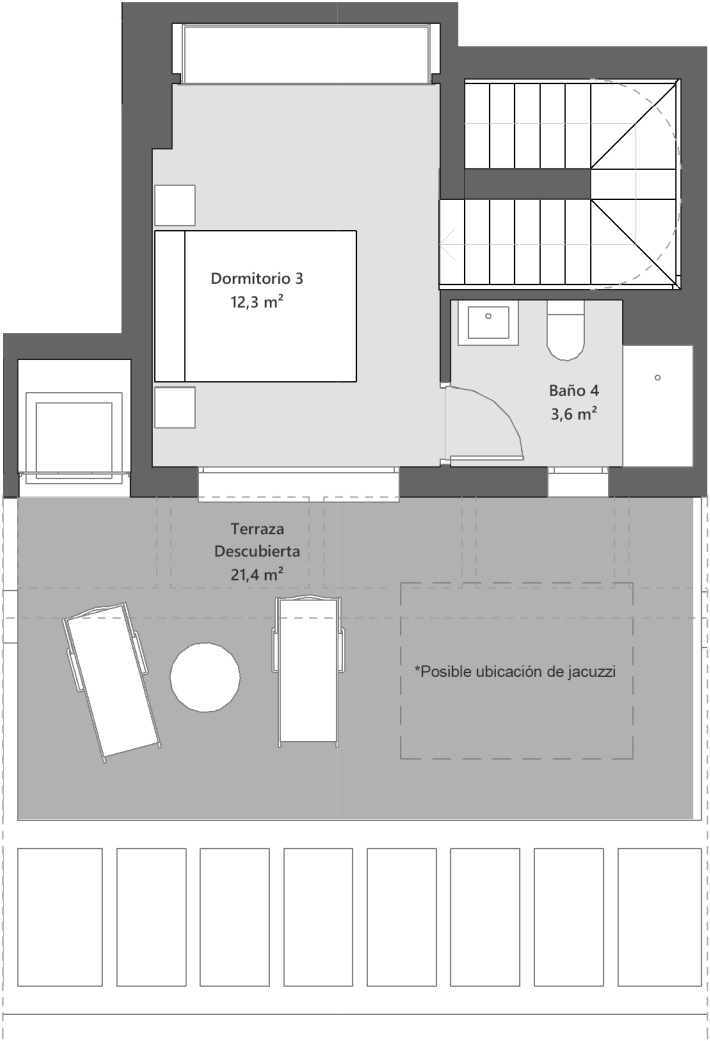
Planta ático
