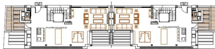
PLANTA ACCESO
