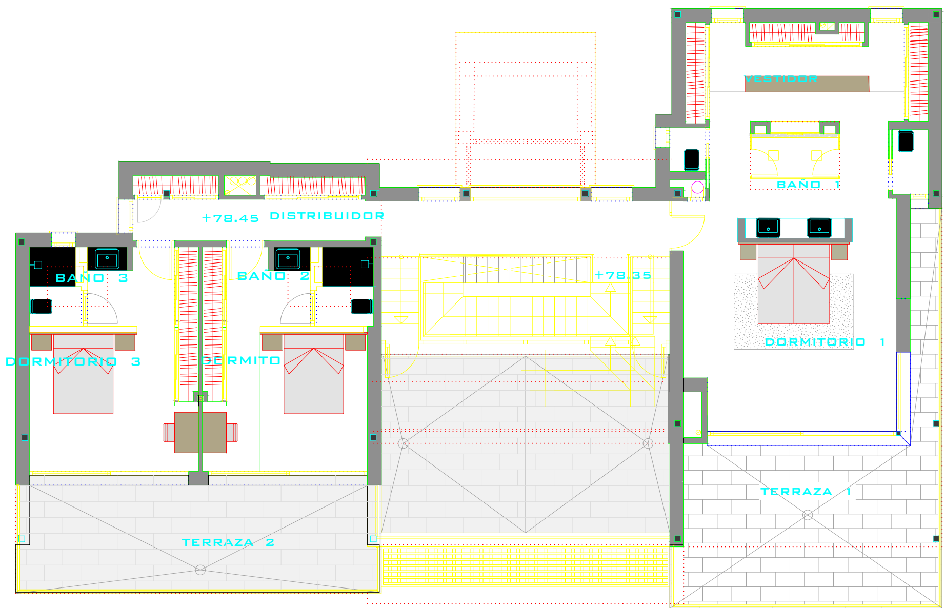
PLANTA ALTA
