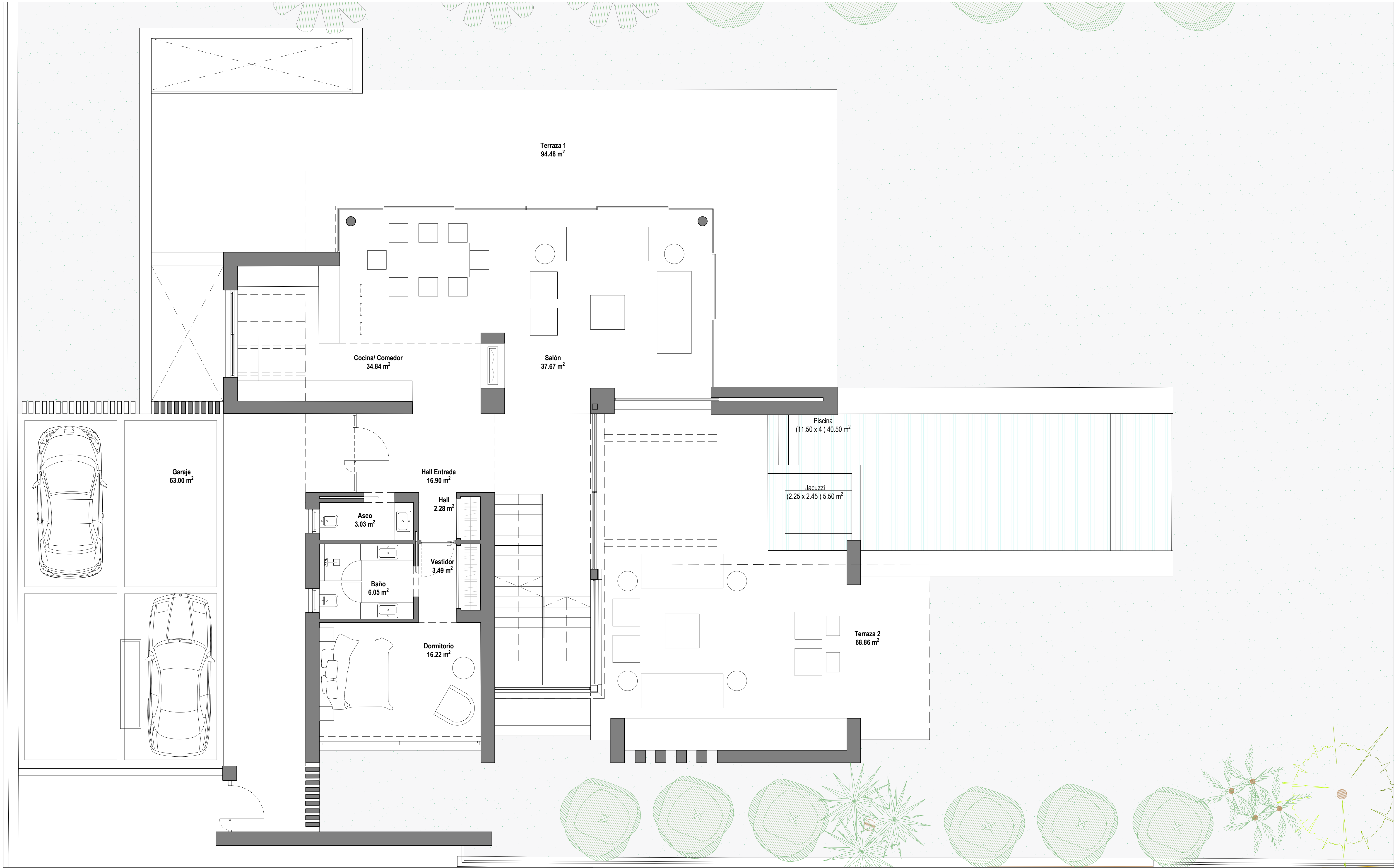
PLANTA BAJA_E:1.50
